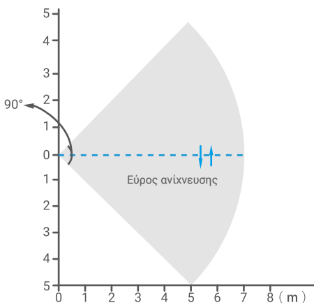
Εικ. 2 Επάνω όψη του εύρους ανίχνευσης
