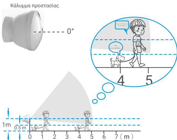
Εικ. 1 Πλαϊνή όψη του εύρους ανίχνευσης
