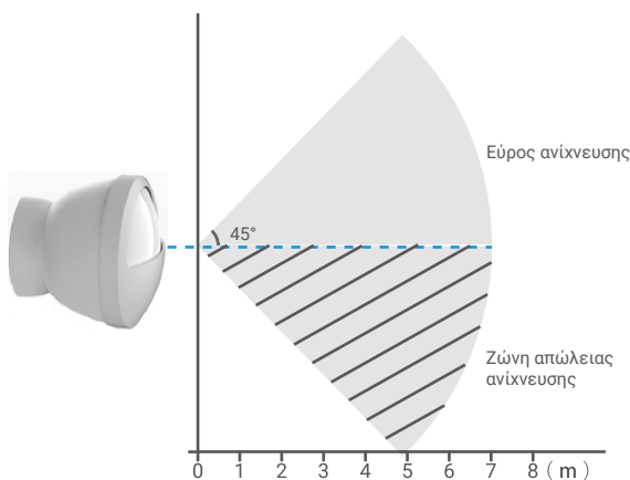
Εικ. 2 Επάνω όψη του εύρους ανίχνευσης
