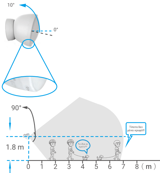
Εικ. 1 Πλαϊνή όψη του εύρους ανίχνευσης
